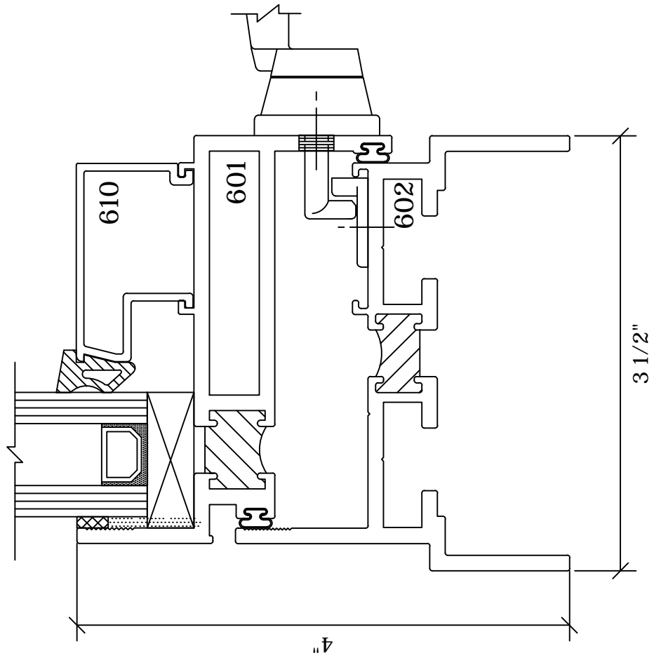
4 RIGHT JAMB 6E5
