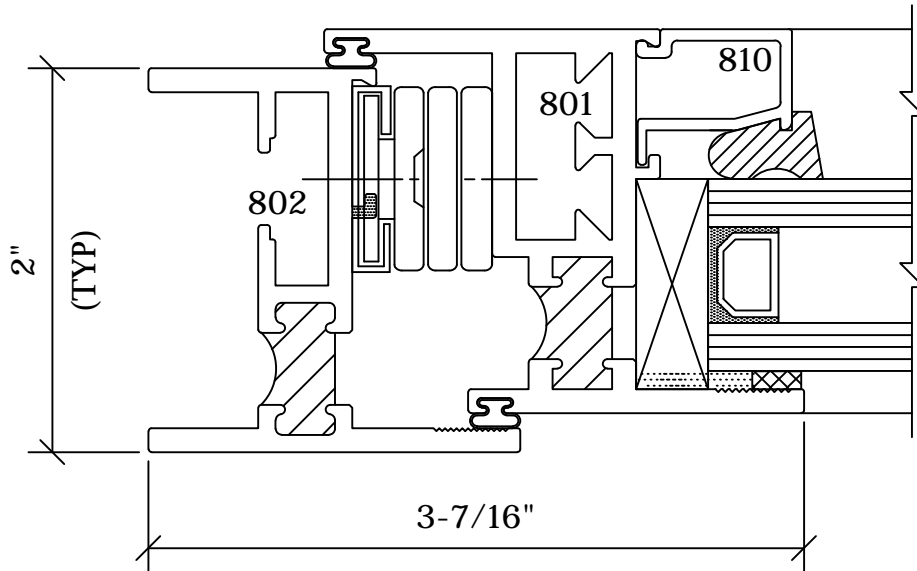
3 JAMB 8B2
