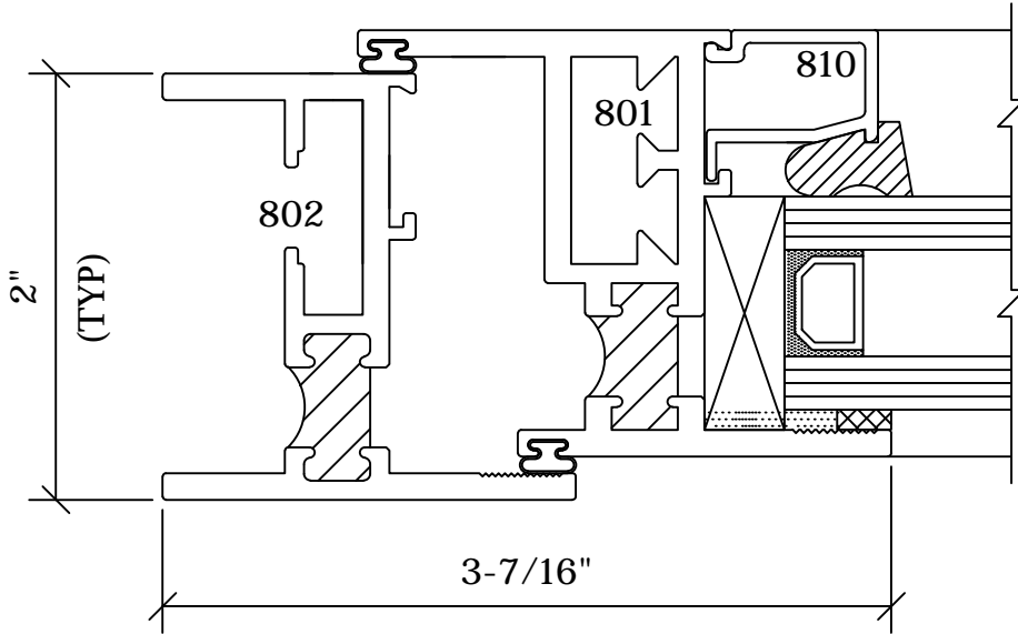
3 LEFT JAMB 8E2
