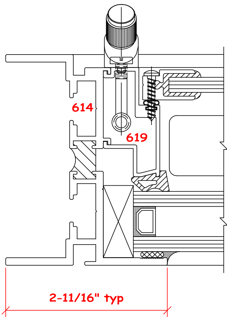
LEFT JAMB - 1" BLIND 12
