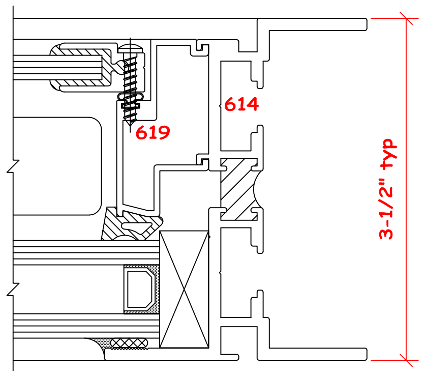
13 RIGHT JAMB - 1" BLIND
