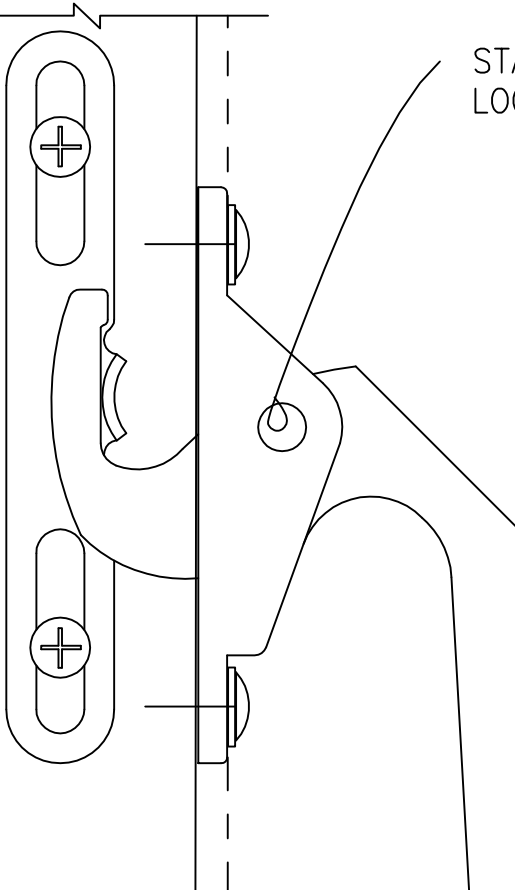
2 Jamb Section B1
